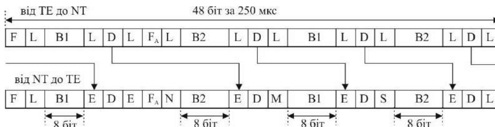
Рис. 6. Структура кадру номінального доступу до ISDN: F – біт кадрування; L – біт компенсації; E – ехо-біт D – каналу; A – біт активації; FA – допоміжний біт кадрування; N – значення протилежне FA; M – багатоканальний біт; B1 – біти B-каналу (16 на кадр); B2 – біти B-каналу (16 на кадр); D – біти D-каналу (4 на кадр); S – резервні біти; E – біт розділення конфлікту
