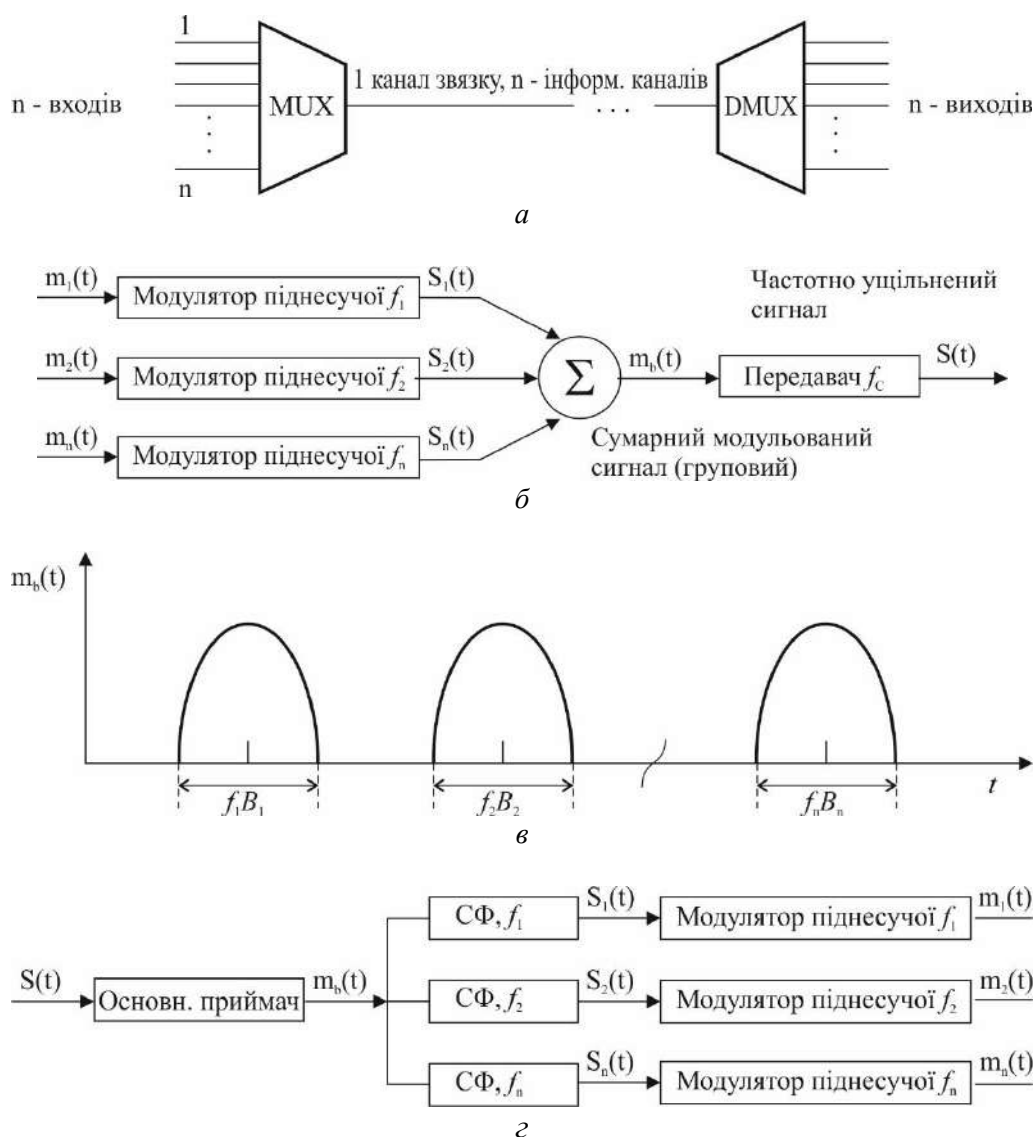
Рис. 3. Система передачі з частотним ущільненням: а – пристрій ущільнення; б – передавач; в – спектр групового сигналу; г – приймач
